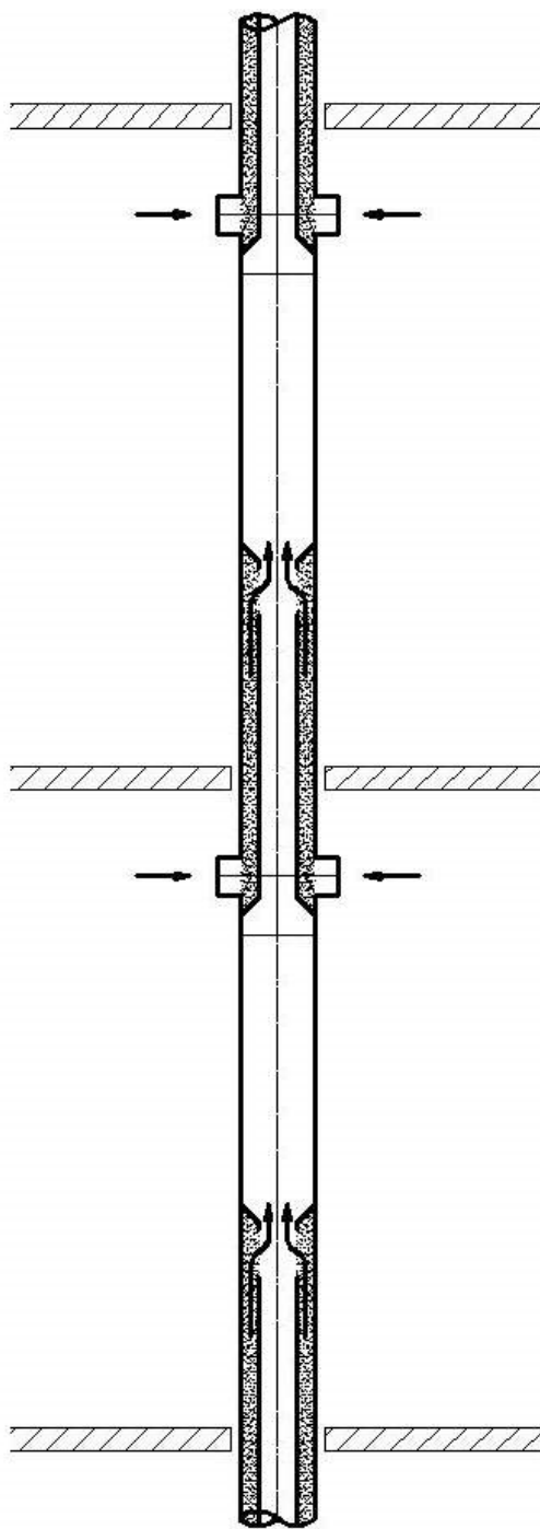
rendszer-összeállítás szintenkénti két csatlakozással
